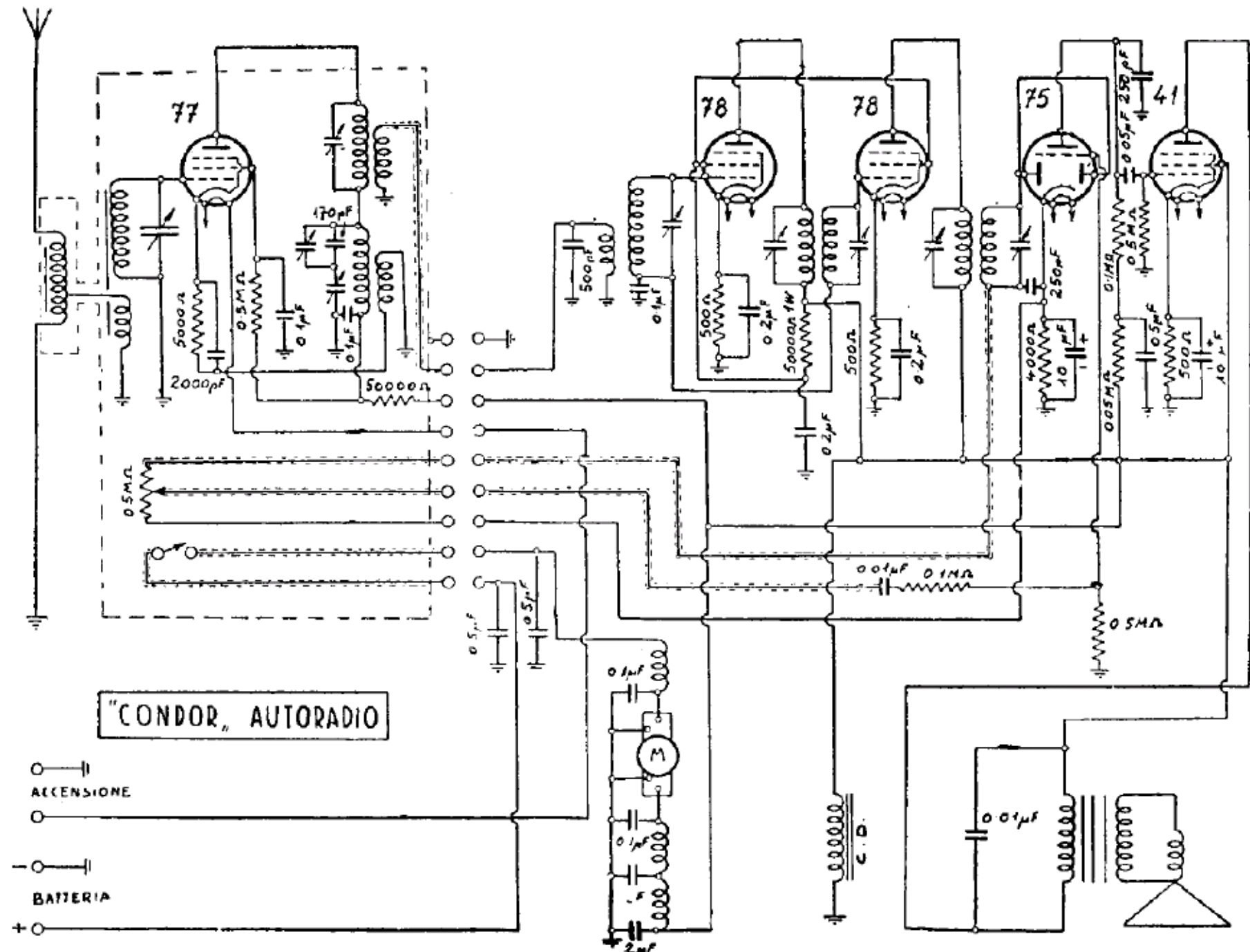
GALLO. — Mod. « Condor ». — Ricevitore autoradio. — Produzione 1937.
